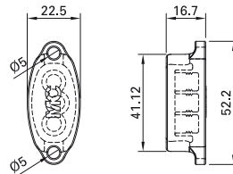
PV-BVK-EVO AC
