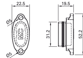
PV-SVK-EVO AC
